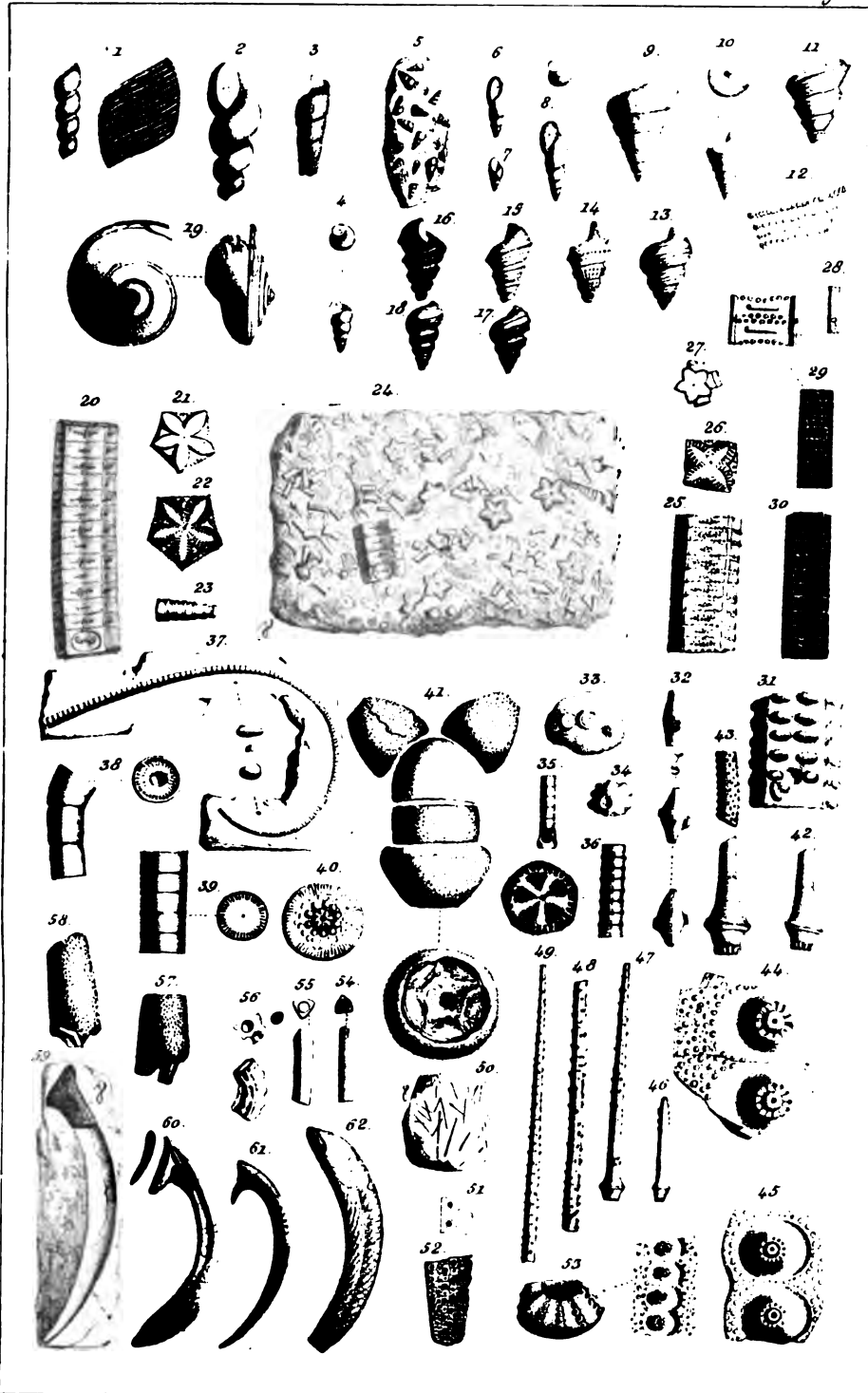
Amnstadt, Jura.
